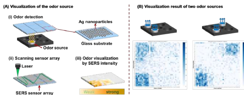
図 4 (A-i) 化学方法で制作した Ag ナノ粒子をガラス基板に堆積して SERS センサを制作した。(A-ii) ガスが吸着した SERS センサアレイをスキャンすると、ガス源を可視化する。(B) 2 つのガス源の可視化結果。
